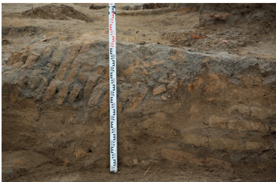
Рис. 3. Забутовка основания башни сырцовыми кирпичами.
